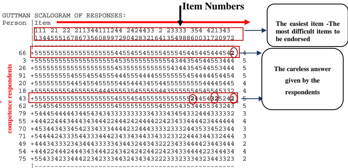
Fig. 5 Guttman Scalogram
